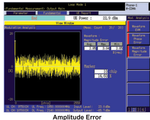
Amplitude Error
